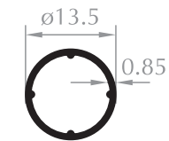
14'LÜK BORU 14 PIPE PROFILE Kod/Code :PD1007 Ağırlık/Weight:0,96 kg/m
