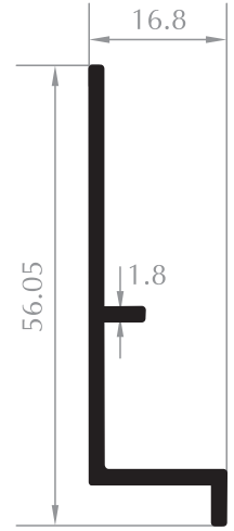
PERVAZ PROFİLİ SILL PROFILE Kod/Code :CE4032 Ağırlık/Weight: 0,370 kg/m
