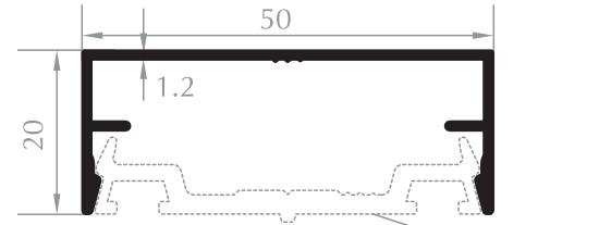
KAPAK PROFİLİ CAP PROFILE Kod/Code :CE3035 Ağırlık/Weight:0,332 kg/m
