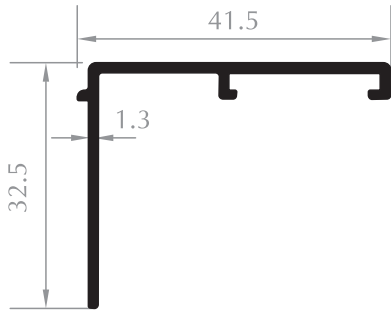
PERVAZ PROFİLİ SILL PROFILE Kod/Code :CE3028 Ağırlık/Weight:0,294 kg/m
