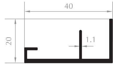
20x40 F PROFİL 20x40 F PROFILE Kod/Code :CE4002 Ağırlık/Weight:0,336 kg/m
