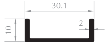
10x30 U PROFİLİ 10x30 U PROFILE Kod/Code :CE4004 Ağırlık/Weight:0,208 kg/m
