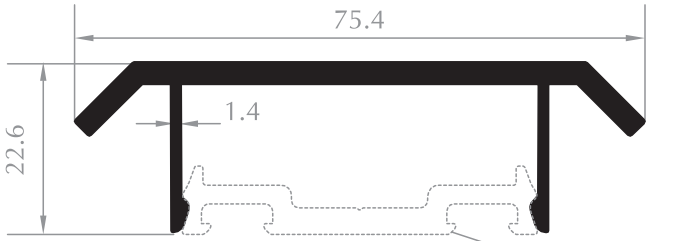
KAPAK PROFİLİ CAP PROFILE Kod/Code :CE3033 Ağırlık/Weight:0,813 kg/m
