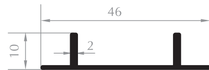
46x10 KANATLI U PROFİLİ 46x10 U PROFILE Kod/Code :CE4003 Ağırlık/Weight:0,297 kg/m
