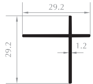
KÖŞE PROFİLİ CORNER PROFILE
