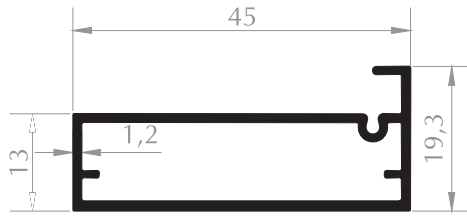
KUTU PROFİLİ BOX PROFILE Kod/Code : MB3034 Ağırlık/Weight : 0,440 kg/m
