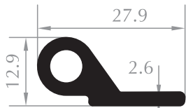
MENTEŞE PROFİLİ HINGE PROFILE Kod/Code :MB1015 Ağırlık/Weight:0,354 kg/m
