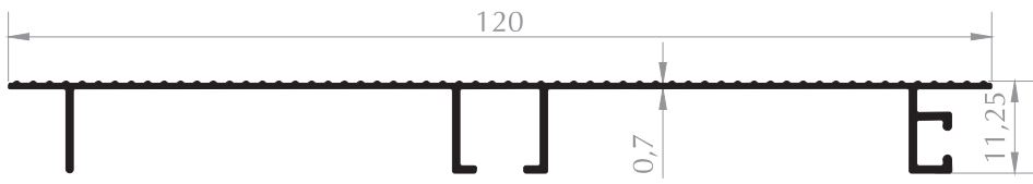
BAZA PROFİLİ BASE PROFILE Kod/Code :MB1049 Ağırlık/Weight:0,388 kg/m
