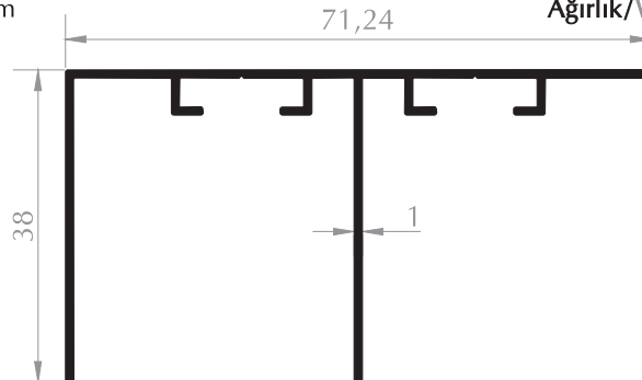
ÜST RAY PROFİLİ TOP RAIL PROFILE Kod/Code :MB1019 Ağırlık/Weight:0,572 kg/m
