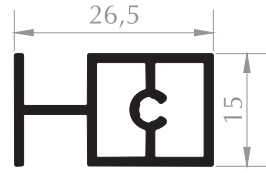
SÜRGÜ DOLAP PROFİLİ SLIDING WARDROBE PROFILE Kod/Code :MB1063 Ağırlık/Weight:0,325 kg/m
