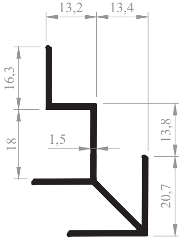
CEPHE KUYRUKLU KÖŞE CORNER PROFILE
