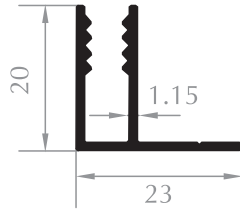
F PROFİLİ F PROFILE Kod/Code :CE2512 Ağırlık/Weight :0,211 kg/m
