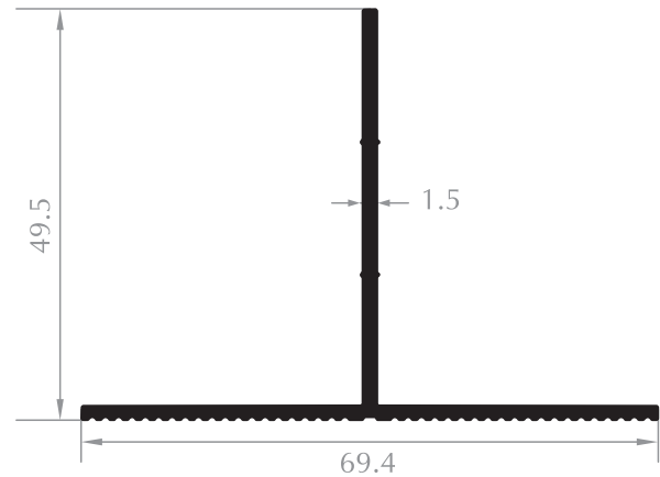
TIRTIKLİ T T PROFILE Kod/Code :CE1407 Ağırlık/Weight:0,451 kg/m
