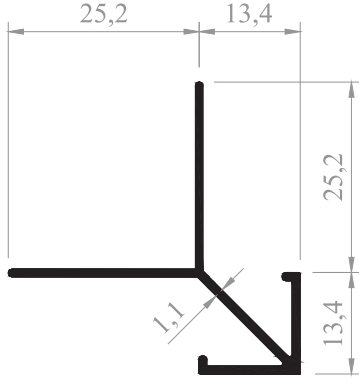
7'LİK KÖŞE ÇITASI CORNER PROFILE
