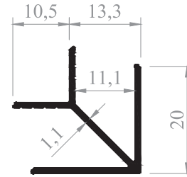
TAŞ GİRİŞ KÖŞE PROFİLİ CORNER PROFILE
