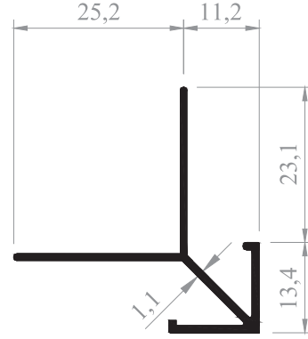
10'LUK KÖŞE ÇITASI CORNER PROFILE
