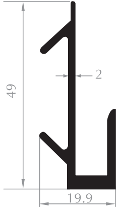
AYARLI KLİPS CLIPS
