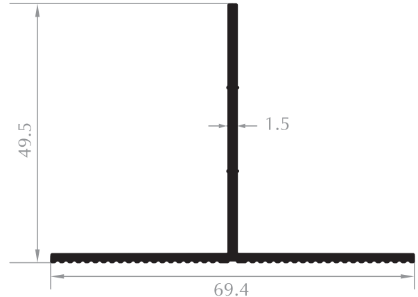
TIRTIKLİ T T PROFILE
