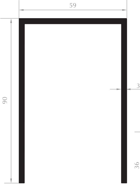
KOMPOZİT U PROFİLİ COMPOSITE U PROFILE Kod/Code : CE2504 Ağırlık/Weight: 1,895 kg/m
