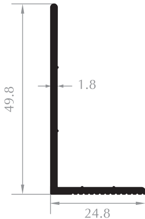
TIRTIKLI L L PROFILE Kod/Code :CE1404 Ağırlık/Weight:0,350 kg/m
