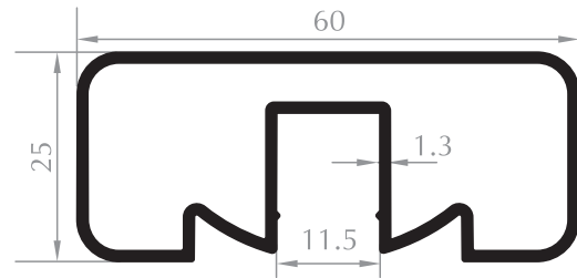
KANALLI ÜST PROFİL SINGLE CHANNEL UPPER PROFILE Kod/Code : KP1018 Ağırlık/Weight : 0.716 kg/m
