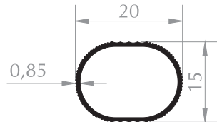
TIRTIKLI BORU PROFİLİ PIPE PROFILE Kod/Code : MB1027 Ağırlık/Weight : 0,114 kg/m
