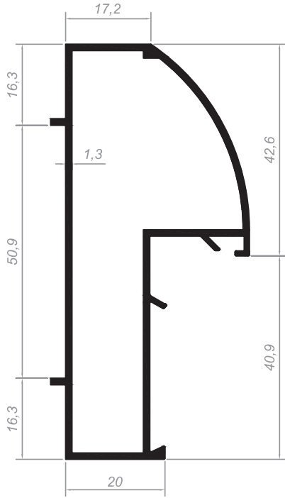
KASA PROFİLİ FRAME PROFILE Kod/Code : OB-F04 Ağırlık/Weight : 0,865 kg/m
