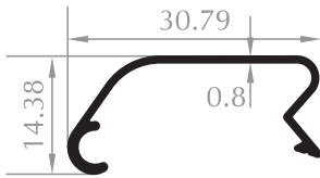
31'LİK ÇERÇEVE PROFİLİ FRAME PROFILE Kod/Code :RK1003 Ağırlık/Weight:0,136 kg/m
