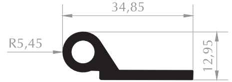
MENTEŞE PROFİLİ HINGE PROFILE Kod/Code : MB1016 Ağırlık/Weight : 0,393 kg/m
