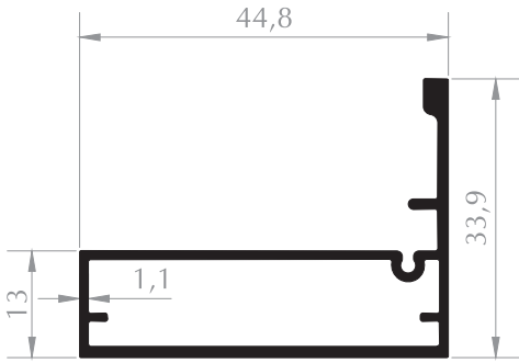
KUTU PROFİLİ BOX PROFILE Kod/Code : MB3033 Ağırlık/Weight : 0,488 kg/m
