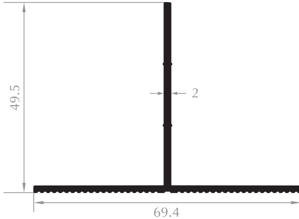
TIRTIKLI T T PROFILE Kod/Code :CE1401 Ağırlık/Weight:0,618 kg/m
