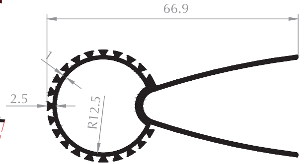
İÇ BAĞLANTI PROFİLİ CONNECTION PROFILE Kod/Code : GK5 Ağırlık/Weight : 0,672 kg/m
