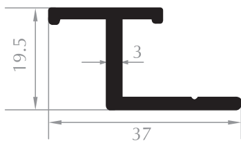
KLİPS CLIPS Kod/Code :CE1007 Ağırlık/Weight:0,425 kg/m
