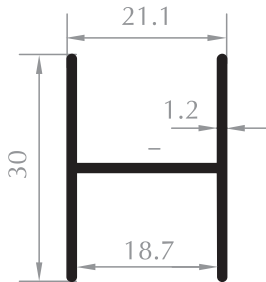
H PROFİLİ H PROFILE Kod/Code : ST5001 Ağırlık/Weight : 0,254 kg/m
