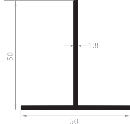
TIRTIKLI T T PROFILE Kod/Code :CE1416 Ağırlık/Weight:0,507 kg/m
