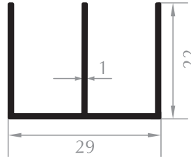
E PROFİLİ E PROFILE Kod/Code :DO1021 Ağırlık/Weight:0,249 kg/m
