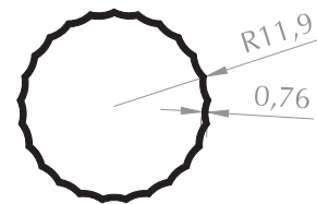
TIRTIKLI BORU PROFİLİ PIPE PROFILE Kod/Code : MB1029 Ağırlık/Weight : 0,152 kg/m
