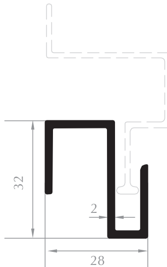
ASKI PROFİLİ HANGER PROFILE Kod/Code :CE2501 Ağırlık/Weight:0,508 kg/m
