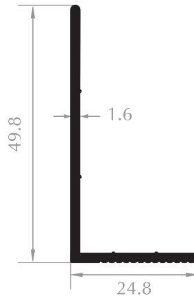
TIRTIKLI L L PROFILE Kod/Code :CE1405 Ağırlık/Weight:0,312 kg/m
