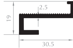
ALT TAŞIYICI PROFİL LOWER PROFILE Kod/Code :CE1006 Ağırlık/Weight:0,349 kg/m
