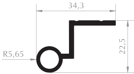
MENTEŞE PROFİLİ HINGE PROFILE Kod/Code : MB1041 Ağırlık/Weight : 0,340 kg/m
