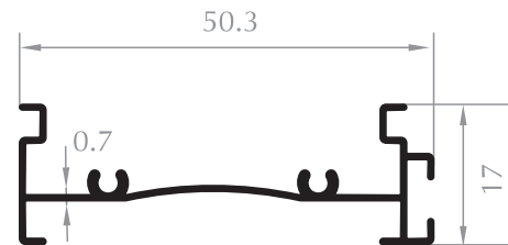
50'LİK ZEBRA KASA 50 FRAME PROFILE Kod/Code : PD1012 Ağırlık/Weight: 0,240 kg/m
