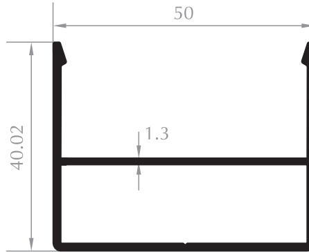
KAPAK PROFİLİ CAP PROFILE Kod/Code :CE4034 Ağırlık/Weight:0,691 kg/m
