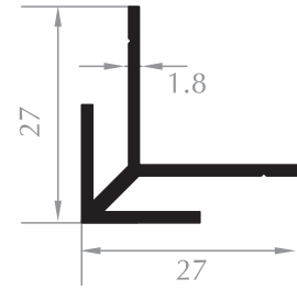
KÖŞE PROFİLİ CORNER PROFILE Kod/Code :CE2508 Ağırlık/Weight:0,283 kg/m
