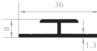
H PROFİLİ H PROFILE Kod/Code :CE2511 Ağırlık/Weight:0,225 kg/m
