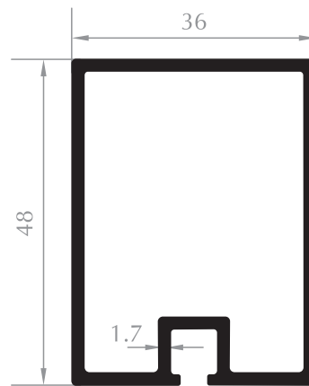
KUTU PROFİLİ BOX PROFILE Kod/Code :CE4033 Ağırlık/Weight: 0,862 kg/m
