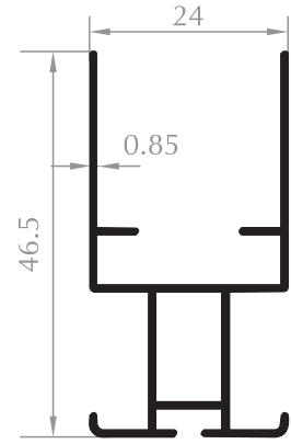
PLİSE KANAT SASH PROFILE
