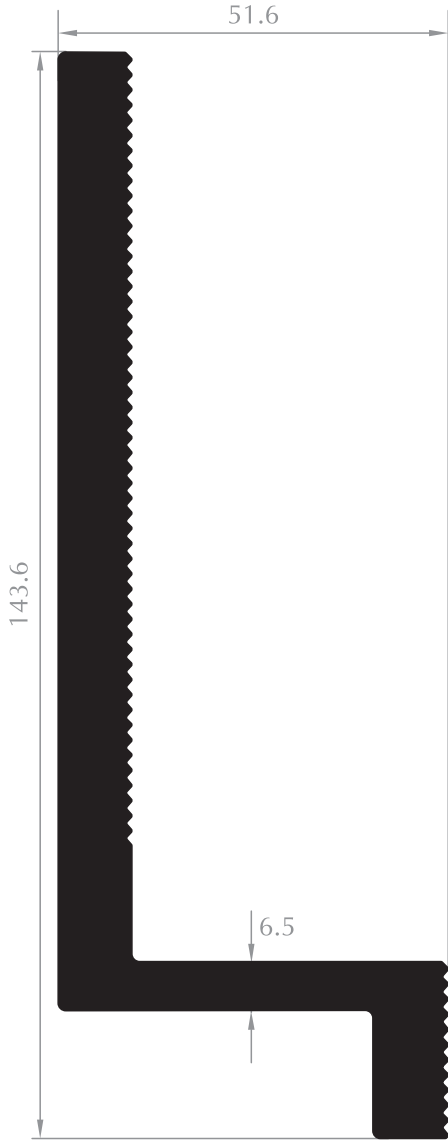
TIRTIKLİ KÖŞEBENT PROFİLİ BRACKET PROFILE Kod/Code :MH1964 Ağırlık/Weight:4,415 kg/m
