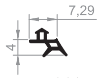
CAM FİTİLİ GASKET
