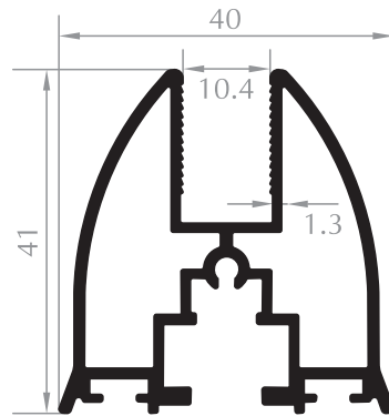
CAM BALKON KANAT SASH PROFILE Kod/Code :CB2010 Ağırlık/Weight :0,791 kg/m
