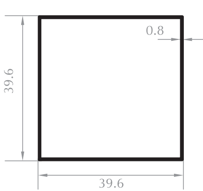
40x40 KUTU PROFİLİ 40x40 BOX PROFILE Kod/Code :ST1036 Ağırlık/Weight:0,331 kg/m
