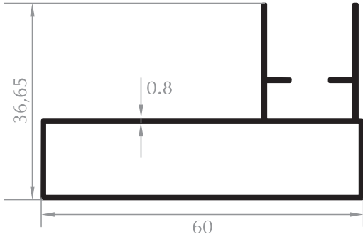
PLİSE KASA 60'LİK FRAME PROFILE Kod/Code : SN2044 Ağırlık/Weight : 0,458 kg/m
