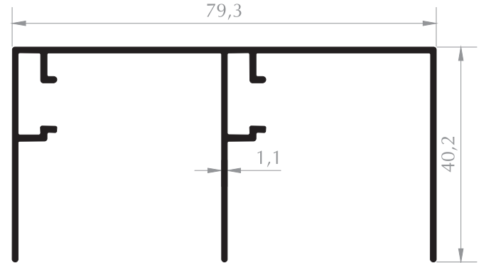
ÜST RAY PROFİLİ TOP RAIL PROFILE Kod/Code :MB1032 Ağırlık/Weight:0,691 kg/m
