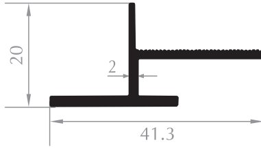
ÜST TAŞIYICI PROFİL UPPER PROFILE Kod/Code :CE1002 Ağırlık/Weight:0,377 kg/m
