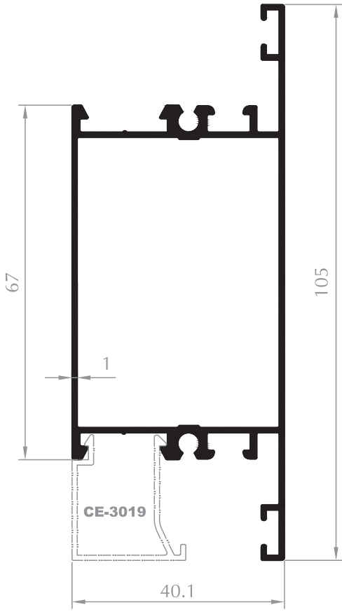
ORTA KAYIT PROFİLİ MULLION PROFILE Kod/Code : CE3016 Ağırlık/Weight: 0,951 kg/m
