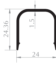
KAPAK PROFİLİ CAP PROFILE
