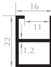
10'LÜK CAMA GÖRE KUTU BOX PROFILE FOR 10mm GLASS Kod/Code : KP1020 Ağırlık/Weight : 0,240 kg/m
