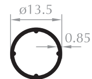
14'LÜK BORU 14 PIPE PROFILE Kod/Code : PD1007 Ağırlık/Weight : 0,96 kg/m
