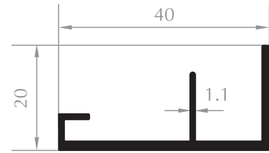
20x40 F PROFİL 20x40 F PROFILE
