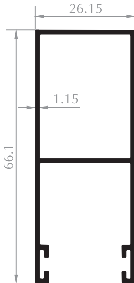
65'LİK DİKME PROFİLİ 65 VERTICAL PROFILE Kod/Code :PJ1019 Ağırlık/Weight:0,615 kg/m
