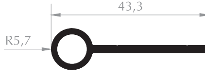
CERMAN MENTEŞE DÜZ HINGE PROFILE Kod/Code : MB1009 Ağırlık/Weight : 0,313 kg/m
