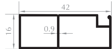
17x42 SİNEKLİK PROFİLİ 20x40 FLYSCREEN PROFILE Kod/Code : SN1003 Ağırlık/Weight : 0,337 kg/m
