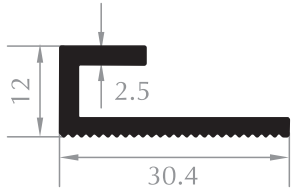
ORTA ASKI PROFİL DÜZ MIDDLE HANGER PROFILE Kod/Code :CE1010 Ağırlık/Weight:0,315 kg/m
