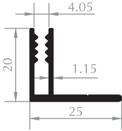
F PROFİLİ F PROFILE Kod/Code :CE2524 Ağırlık/Weight:0,258 kg/m
