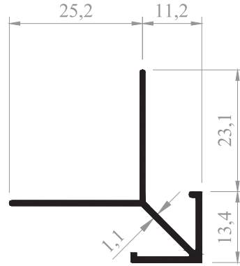
10'LUK KÖŞE ÇITASI CORNER PROFILE Kod/Code : CE1409 Ağırlık/Weight : 0,270 kg/m
