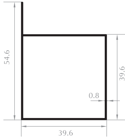
40x40 KULAKLI PROFİL 40x40 BOX PROFILE Kod/Code :MB1017 Ağırlık/Weight:0,368 kg/m
