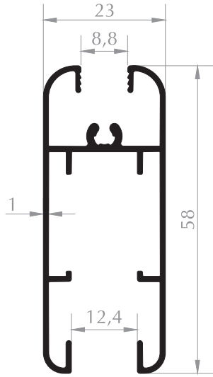
ALT / ÜST BAĞLANTI PROFİLİ BOTTOM / TOP CONNECTION PROFILE Kod/Code : MB1056 Ağırlık/Weight : 0,545 kg/m
