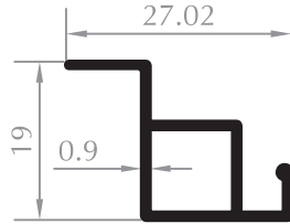
SİNEKLİK PROFİLİ FLYSCREEN PROFILE Kod/Code :SN2050 Ağırlık/Weight :0,174 kg/m
