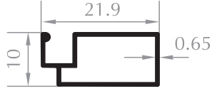
10x20 PENCERE SİNEKLİK 10x20 FLYSCREEN FOR WINDOW Kod/Code : SN1001 Ağırlık/Weight : 0,116 kg/m
