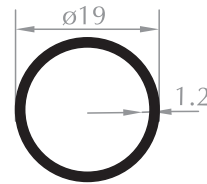
19'LUK BORU Ø19 PIPE Kod/Code : ST3005 Ağırlık/Weight : 0,182 kg/m
