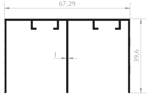
ÜST RAY PROFİLİ TOP RAIL PROFILE Kod/Code :MB1030 Ağırlık/Weight:0,552 kg/m
