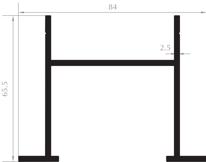
KOMPOZİT ASKI PROFİLİ COMPOSITE HANGER PROFILE Kod/Code : CE4023 Ağırlık/Weight: 1,468 kg/m
