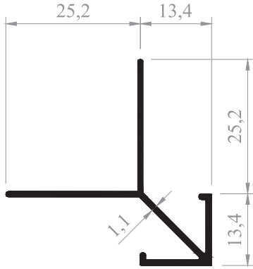
7'LİK KÖŞE ÇITASI CORNER PROFILE Kod/Code : CE1408 Ağırlık/Weight : 0,275 kg/m
