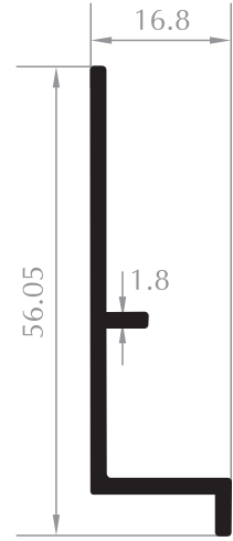
PERVAZ PROFİLİ SILL PROFILE Kod/Code :CE4032 Ağırlık/Weight: 0,370 kg/m
