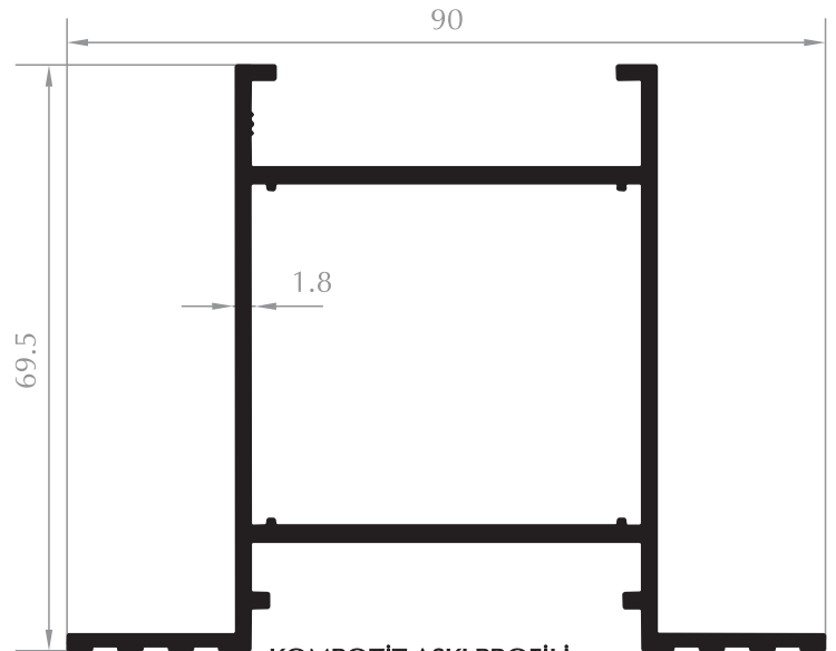
KOMPOZİT ASKI PROFİLİ COMPOSITE HANGER PROFILE Kod/Code : CE2503 Ağırlık/Weight: 1,434 kg/m
