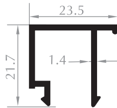
TEK CAM ÇİTASI GLAZING BEAD Kod/Code :DO1008 Ağırlık/Weight:0,268 kg/m
