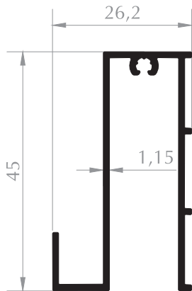
SÜRGÜ DOLAP PROFİLİ SLIDING WARDROBE PROFILE Kod/Code :MB1060 Ağırlık/Weight:0,425 kg/m
