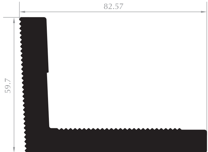
TIRTIKLİ KÖŞEBENT PROFİLİ BRACKET PROFILE Kod/Code :MH1967 Ağırlık/Weight:3,711 kg/m
