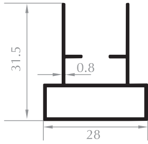
PLİSE KASA 28'LİK FRAME PROFILE Kod/Code : SN2035 Ağırlık/Weight : 0,271 kg/m
