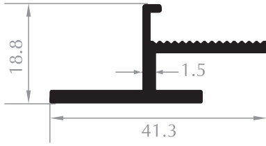
ÜST TAŞIYICI PROFİL UPPER PROFILE Kod/Code :CE1001 Ağırlık/Weight:0,396 kg/m
