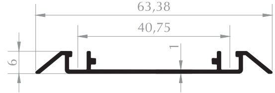
ALT RAY PROFİLİ RAIL PROFILE Kod/Code : MB3019 Ağırlık/Weight : 0,252 kg/m
