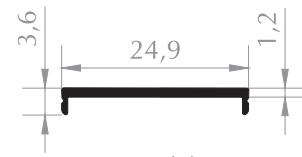
KAPAK PROFİLİ (MB1061) CAP PROFILE Kod/Code : MB1062 Ağırlık/Weight : 0,089 kg/m
