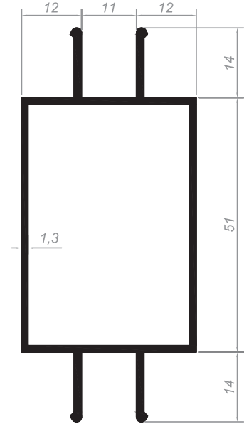
KASA PROFİLİ FRAME PROFILE Kod/Code : OB-F01 Ağırlık/Weight : 0,821 kg/m
