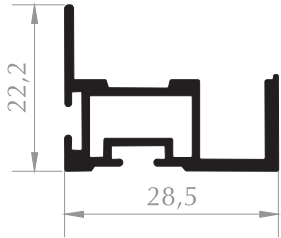
SÜRGÜ DOLAP PROFİLİ SLIDING WARDROBE PROFILE Kod/Code :MB1059 Ağırlık/Weight:0,352 kg/m
