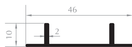
46x10 KANATLI U PROFİLİ 46x10 U PROFILE
