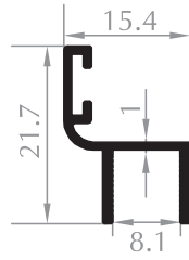
KÜÇÜK H PROFİLİ H PROFILE Kod/Code :CB3005 Ağırlık/Weight:0,152 kg/m
