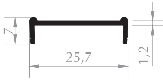
KAPAK PROFİLİ CAP PROFILE Kod/Code : MB3002 Ağırlık/Weight : 0,122 kg/m
