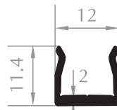
DERZ ÇİTA PROFİLİ JOINT PROFILE Kod/Code :CE4016 Ağırlık/Weight:0,116 kg/m
