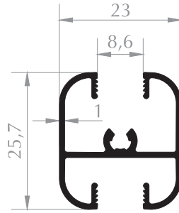
ORTA BAĞLANTI PROFİLİ MIDDLE CONNECTION PROFILE Kod/Code : MB1047 Ağırlık/Weight : 0,314 kg/m
