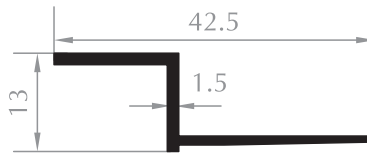
FAYANS ÇİTASI TILE PROFILE Kod/Code :MH1007 Ağırlık/Weight:0,188 kg/m
