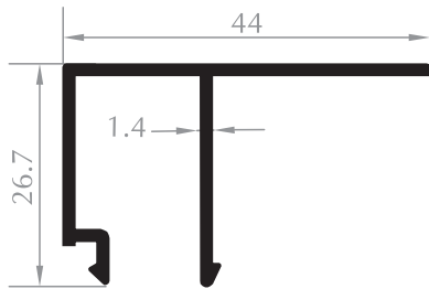
TEK CAM ÇİTASI GLAZING BEAD Kod/Code :DO1009 Ağırlık/Weight:0,380 kg/m
