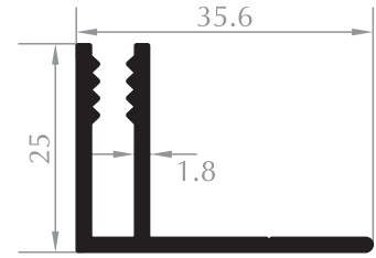
F PROFİLİ F PROFILE Kod/Code :CE2518 Ağırlık/Weight:0,423 kg/m
