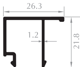
TEK CAM ÇİTASI GLAZING BEAD Kod/Code :DO1016 Ağırlık/Weight:0,232 kg/m
