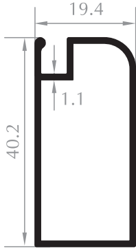
20x40 KAPI SİNEKLİĞİ 20x40 FLYSCREEN FOR DOOR Kod/Code : SN1005 Ağırlık/Weight : 0,359 kg/m
