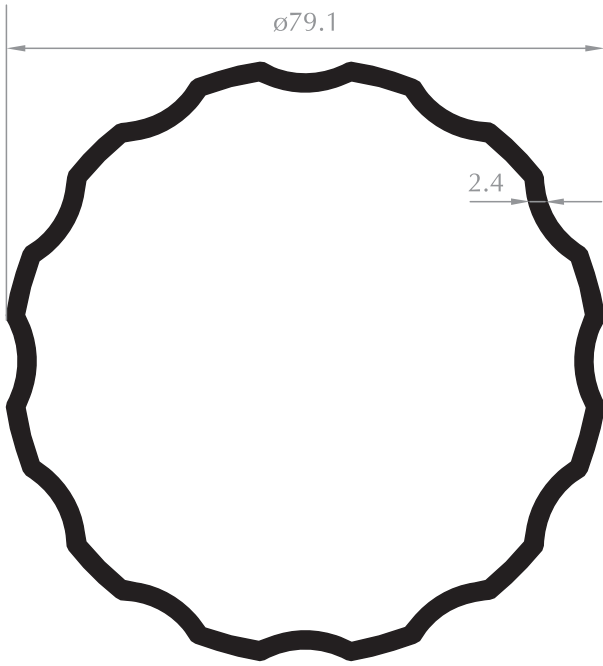
80'LİK YIVLİ BORU PROFİLİ STOVE PIPE Kod/Code :MH1957 Ağırlık/Weight:1,620 kg/m
