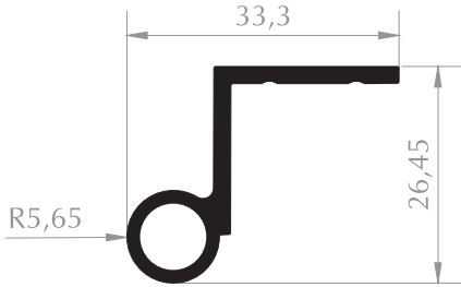
MENTEŞE PROFİLİ HINGE PROFILE Kod/Code : MB1042 Ağırlık/Weight : 0,361 kg/m
