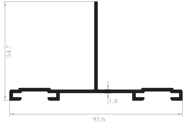
ÇİFT KANALLI T DOUBLE CHANNEL PROFILE Kod/Code : CE1606 Ağırlık/Weight: 0,890 kg/m
