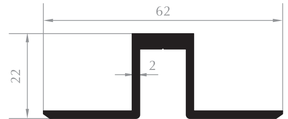
OMEGA PROFİL OMEGA PROFILE Kod/Code :CE4014 Ağırlık/Weight:0,610 kg/m
