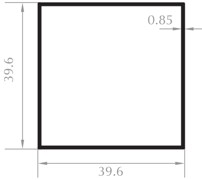
40x40 KUTU PROFİLİ 40x40 BOX PROFILE Kod/Code :ST1018 Ağırlık/Weight:0,357 kg/m
