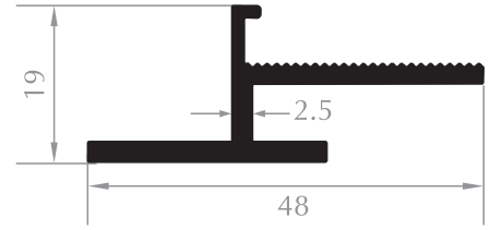
ÜST TAŞIYICI PROFİL UPPER PROFILE Kod/Code :CE1003 Ağırlık/Weight:0,470 kg/m
