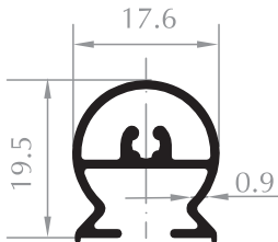
ÖN DİKME VERTICAL FRONT STRUT Kod/Code :DK1010 Ağırlık/Weight:0,221 kg/m
