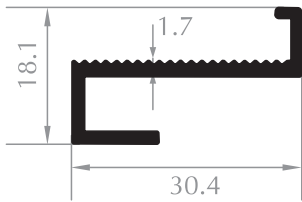
ALT TAŞIYICI PROFİL LOWER PROFILE Kod/Code :CE1004 Ağırlık/Weight:0,283 kg/m
