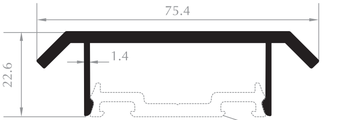
KAPAK PROFİLİ CAP PROFILE
