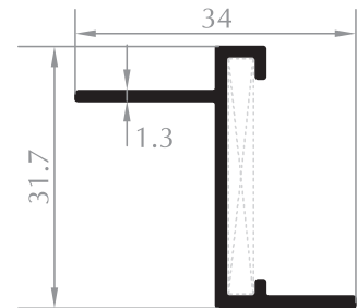
KOMPOZİT ASKI COMPOSITE HANGER PROFILE Kod/Code :CE2523 Ağırlık/Weight:0,269 kg/m
