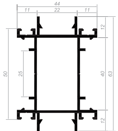
KASA PROFİLİ FRAME PROFILE Kod/Code : OB-F02 Ağırlık/Weight : 0,982 kg/m
