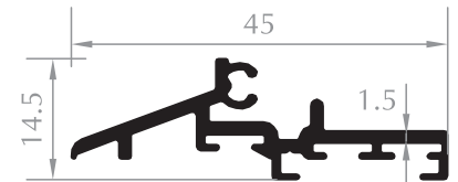
FAYANS ÇİTASI TILE PROFILE Kod/Code :MH1948 Ağırlık/Weight:0,343 kg/m
