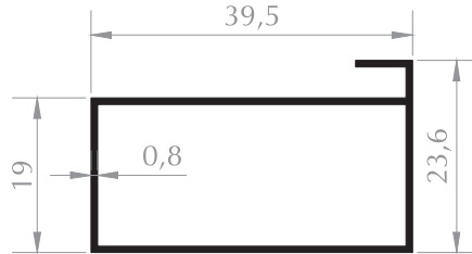
KUTU PROFİLİ BOX PROFILE Kod/Code : MB1021 Ağırlık/Weight : 0,273 kg/m
