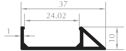
SİNEKLİK PROFİLİ FLYSCREEN PROFILE Kod/Code :SN2048 Ağırlık/Weight :0,193 kg/m
