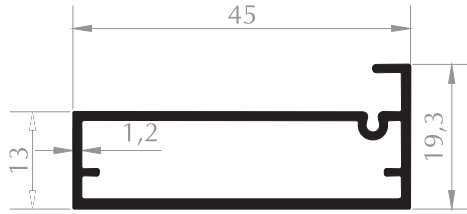
KUTU PROFİLİ BOX PROFILE Kod/Code : MB3034 Ağırlık/Weight : 0,440 kg/m
