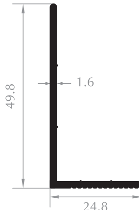
TIRTIKLI L L PROFILE Kod/Code :CE1405 Ağırlık/Weight:0,312 kg/m
