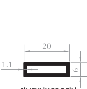
SİNEKLİK PROFİLİ FLYSCREEN PROFILE Kod/Code :SN2046 Ağırlık/Weight :0,142 kg/m
