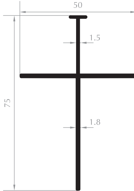
T PROFİLİ T PROFILE Kod/Code :CE1102 Ağırlık/Weight:0,602 kg/m
