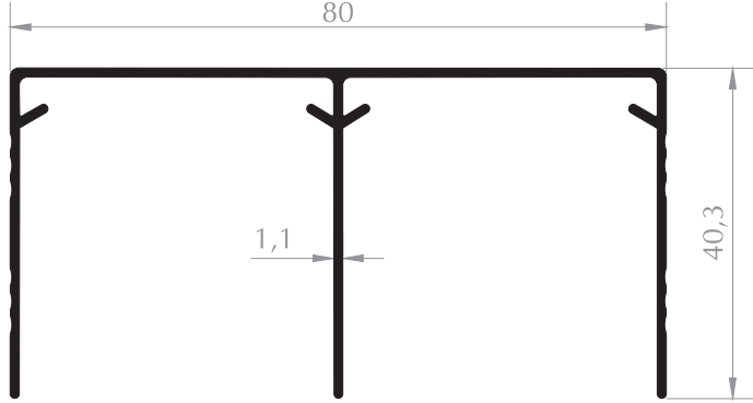
ÜST RAY PROFİLİ TOP RAIL PROFILE Kod/Code :MB3018 Ağırlık/Weight:0,623 kg/m
