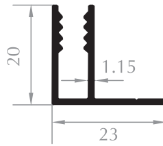
F PROFİLİ F PROFILE Kod/Code :CE2512 Ağırlık/Weight:0,211 kg/m
