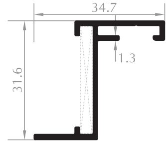
KASET PROFİLİ SASH PROFILE Kod/Code :CE2522 Ağırlık/Weight:0,311 kg/m
