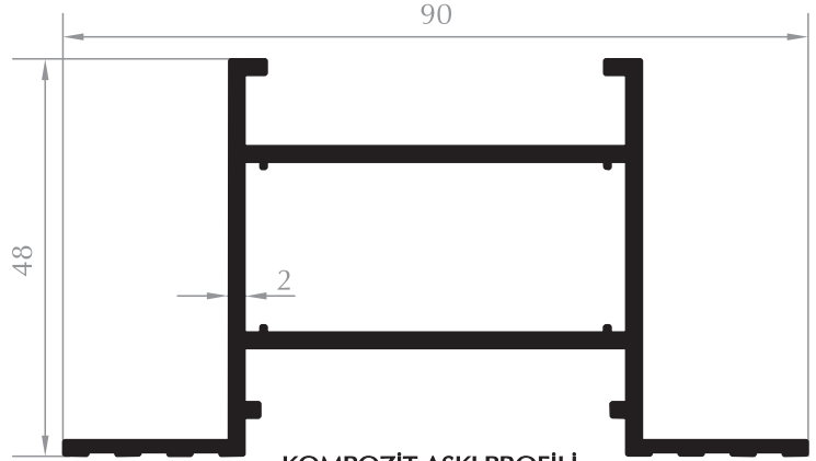
KOMPOZİT ASKI PROFİLİ COMPOSITE HANGER PROFILE Kod/Code : CE2506 Ağırlık/Weight: 1,271 kg/m
