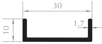
10x30 U PROFİLİ 10x30 U PROFILE Kod/Code :CE4007 Ağırlık/Weight:0,214 kg/m
