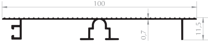
BAZA PROFİLİ BASE PROFILE Kod/Code :MB1048 Ağırlık/Weight:0,385 kg/m
