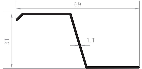
Z PROFİLİ Z PROFILE Kod/Code :MH1934 Ağırlık/Weight:0,276 kg/m
