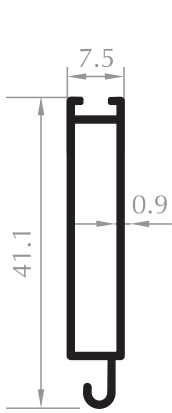
ALT ETEK PROFİLİ LOWER PROFILE Kod/Code :PJ1010 Ağırlık/Weight:0,228 kg/m
