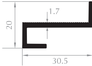
ALT TAŞIYICI PROFİL LOWER PROFILE Kod/Code :CE1005 Ağırlık/Weight:0,264 kg/m
