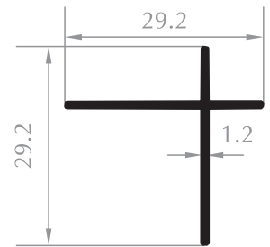
KÖŞE PROFİLİ CORNER PROFILE Kod/Code :CE4021 Ağırlık/Weight:0,187 kg/m
