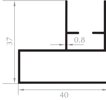
PLİSE KASA 40'LİK FRAME PROFILE Kod/Code : SN2037 Ağırlık/Weight : 0,347 kg/m
