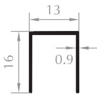
PANJUR DAR U U PROFILE Kod/Code :PJ1017 Ağırlık/Weight:0,105 kg/m
