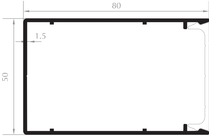
KAPAK PROFİLİ CAP PROFILE
