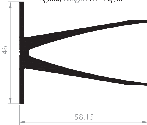
90° BAĞLANTI PROFİLİ 90° CONNECTION PROFILE Kod/Code : GK6 Ağırlık/Weight: 1,114 kg/m
