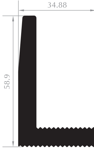
TIRTIKLİ KÖŞEBENT PROFİLİ BRACKET PROFILE Kod/Code :MH1965 Ağırlık/Weight:1,783 kg/m
