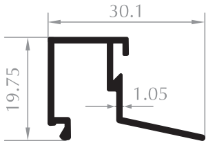
ÇİFT CAM ÇİTASI GLAZING BEAD Kod/Code : DO2008 Ağırlık/Weight : 0,220 kg/m
