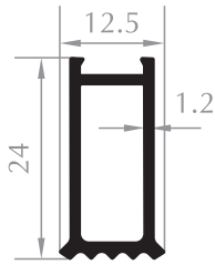
SIYIRICI PROFİL VARIOUS PROFILE Kod/Code :MH1104 Ağırlık/Weight:0,219 kg/m
