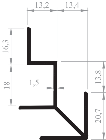
CEPHE KUYRUKLU KÖŞE CORNER PROFILE Kod/Code : CE1412 Ağırlık/Weight : 0,482 kg/m
