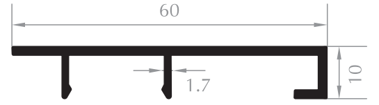
KAPAK PROFİLİ CAP PROFILE Kod/Code : MH1002 Ağırlık/Weight : 0,392 kg/m
