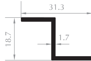
Z PROFİLİ Z PROFILE Kod/Code :CE2507 Ağırlık/Weight:0,222 kg/m
