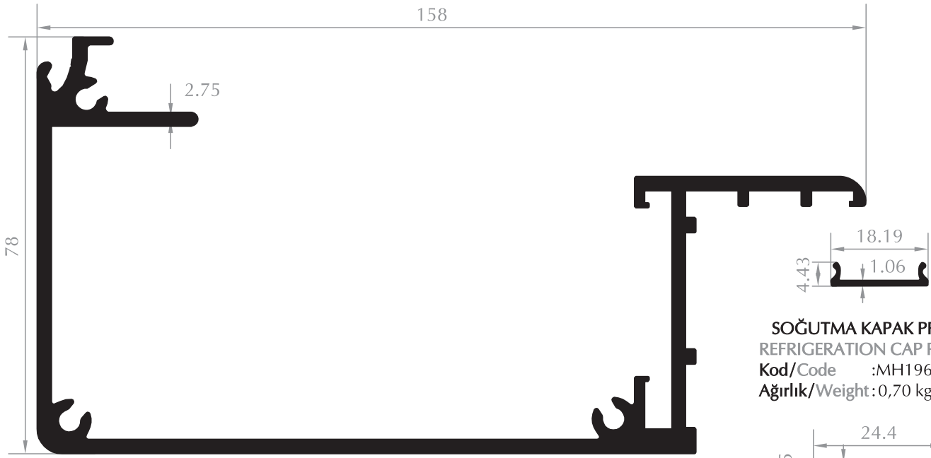
SOĞUTMA PROFİLİ REFRIGERATION PROFILE Kod/Code :MH1919 Ağırlık/Weight: 2,879 kg/m
