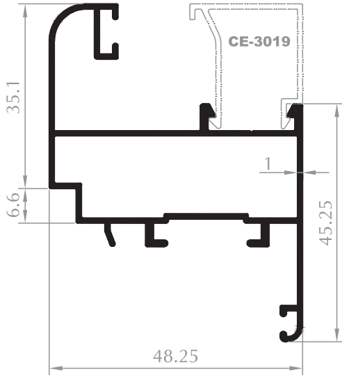
KANAT PROFİLİ SASH PROFILE
