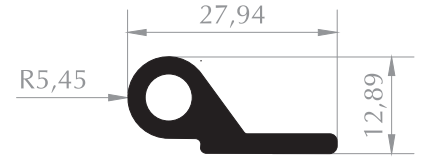
MENTEŞE PROFİLİ HINGE PROFILE Kod/Code : MB1015 Ağırlık/Weight : 0,354 kg/m
