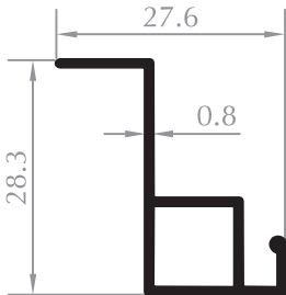
SİNEKLİK PROFİLİ FLYSCREEN PROFILE Kod/Code :SN2052 Ağırlık/Weight :0,180 kg/m
