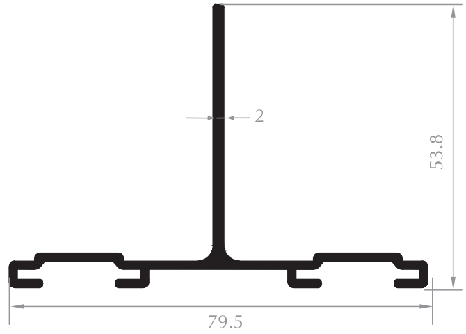
ÇİFT KANALLI T DOUBLE CHANNEL PROFILE Kod/Code : CE1604 Ağırlık/Weight: 0,878 kg/m
