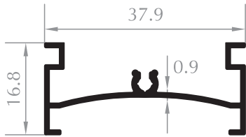
38'LİK KASA 38 FRAME PROFILE Kod/Code : PD1002 Ağırlık/Weight : 0,237 kg/m
