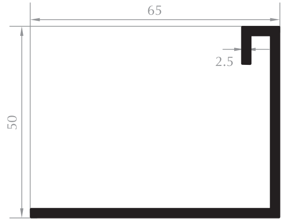
KÖŞEBENT PROFİLİ BRACKET PROFILE Kod/Code :MH1959 Ağırlık/Weight: 0,863 kg/m
