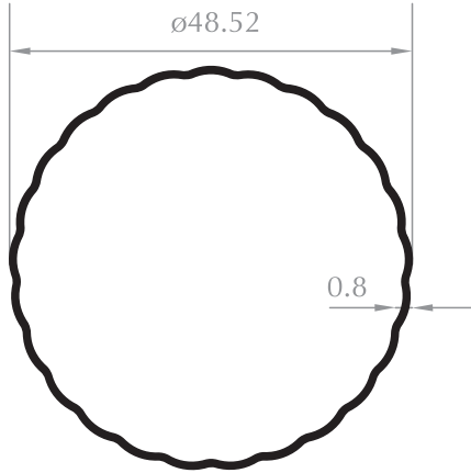
48'LİK SOBA BORUSU STOVE PIPE Kod/Code :MH1928 Ağırlık/Weight:0,328 kg/m
