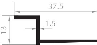
FAYANS ÇİTASI TILE PROFILE Kod/Code :MH1006 Ağırlık/Weight:0,167 kg/m
