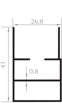
PLİSE KASA FRAME PROFILE
