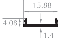
KOMPOZİT BASKI KAPAĞI COMPOSITE CAP PROFILE Kod/Code :CE2510 Ağırlık/Weight:0,076 kg/m
