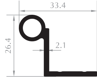
MOBİLYA MENTEŞE HINGE PROFILE Kod/Code :MB1011 Ağırlık/Weight:0,361 kg/m
