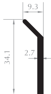
MEMBRAN ÇITASI MEMBRANE PROFILE Kod/Code :CE4010 Ağırlık/Weight:0,245 kg/m
