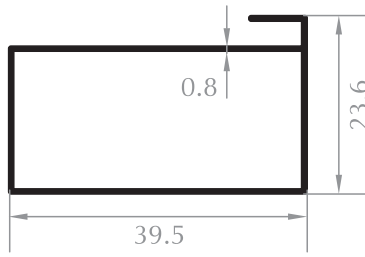
20x40 KUTU PROFİLİ 20x40 BOX PROFILE Kod/Code :MB1021 Ağırlık/Weight:0,273 kg/m
