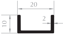
10x20 U PROFİLİ 10x20 U PROFILE Kod/Code :CE4006 Ağırlık/Weight:0,174 kg/m
