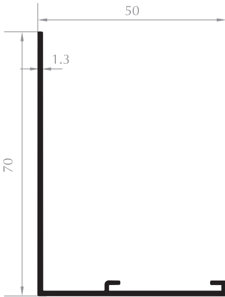
PERVAZ PROFİLİ SILL PROFILE Kod/Code :CE4029 Ağırlık/Weight:0,450 kg/m
