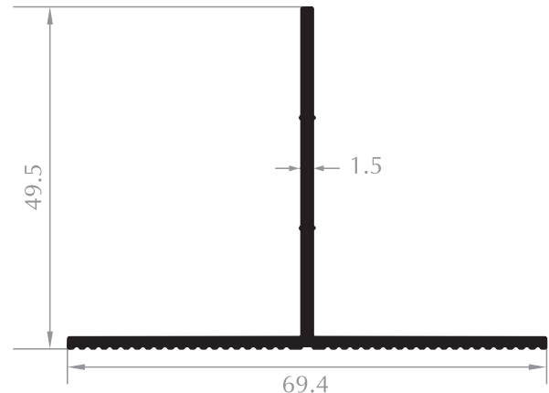
TIRTIKLİ T T PROFILE
