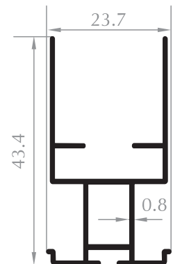
PLİSE KANAT SASH PROFILE
