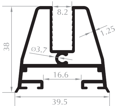
CAM BALKON KANAT SASH PROFILE Kod/Code :CB3002 Ağırlık/Weight:0,751 kg/m
