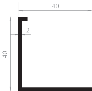
40x40 PERVAZ KÖŞEBENT 40x40 SILL PROFILE Kod/Code :CE4015 Ağırlık/Weight:0,439 kg/m
