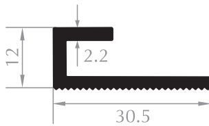
ORTA ASKI PROFİL DÜZ MIDDLE HANGER PROFILE Kod/Code :CE1009 Ağırlık/Weight:0,284 kg/m
