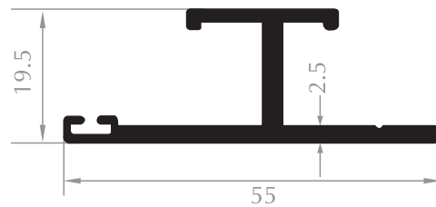
TAŞIYICI KLİPS CLIPS Kod/Code :CE1008 Ağırlık/Weight:0,620 kg/m
