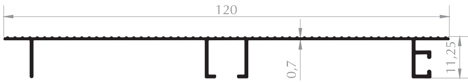
BAZA PROFİLİ BASE PROFILE Kod/Code :MB1049 Ağırlık/Weight:0,388 kg/m
