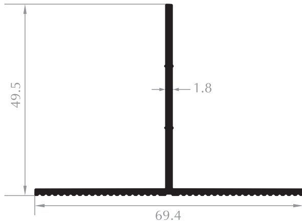
TIRTIKLİ T T PROFILE Kod/Code :CE1406 Ağırlık/Weight:0,545 kg/m
