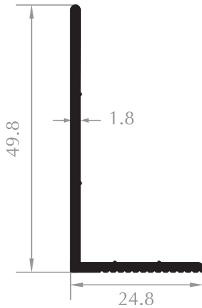
TIRTIKLİ L L PROFILE
