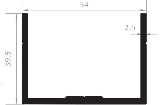
KOMPOZİT BAĞLANTI PROFİLİ COMPOSITE CONNECTION PROFILE Kod/Code : CE4022 Ağırlık/Weight: 0,908 kg/m
