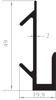
AYARLI KLİPS CLIPS
