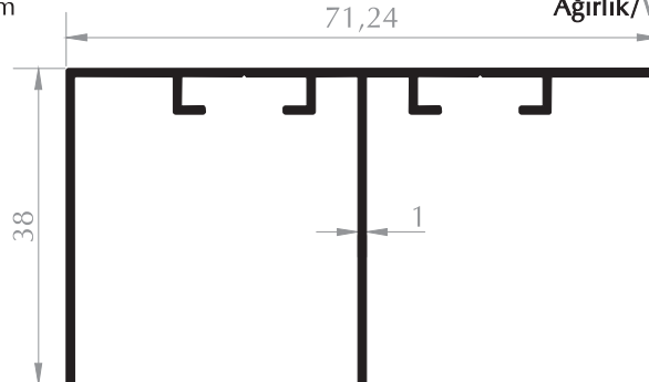
ÜST RAY PROFİLİ TOP RAIL PROFILE Kod/Code :MB1019 Ağırlık/Weight:0,572 kg/m
