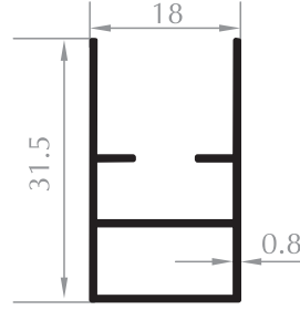
PLİSE KASA 18'LİK FRAME PROFILE Kod/Code : SN2036 Ağırlık/Weight : 0,227 kg/m
