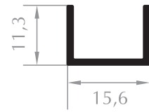
U PROFİLİ U PROFILE Kod/Code :CE1414 Ağırlık/Weight:0,119 kg/m
