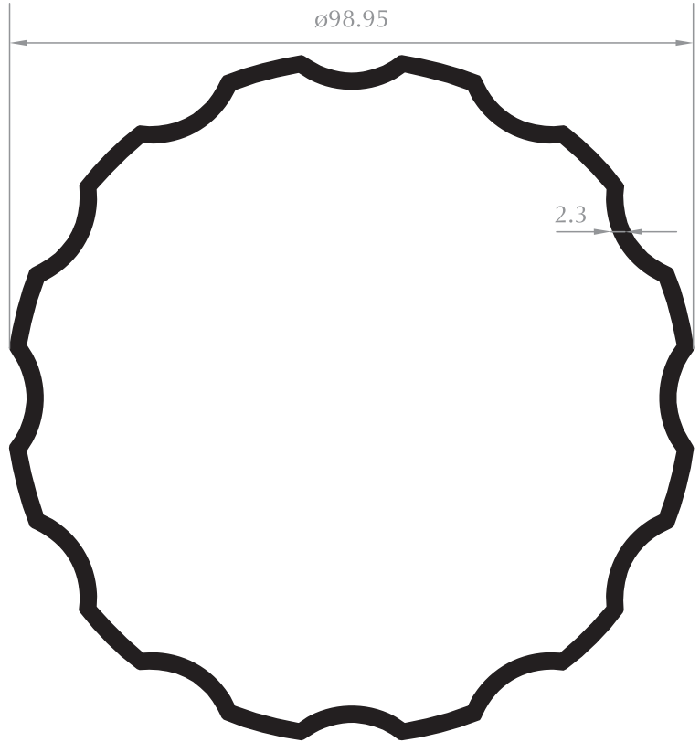
100'LÜK YIVLİ BORU PROFİLİ STOVE PIPE Kod/Code :MH1958 Ağırlık/Weight:1,995 kg/m
