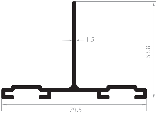
ÇİFT KANALLI T DOUBLE CHANNEL PROFILE Kod/Code : CE1602 Ağırlık/Weight: 0,684 kg/m
