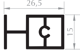
SÜRGÜ DOLAP PROFİLİ SLIDING WARDROBE PROFILE Kod/Code :MB1063 Ağırlık/Weight:0,325 kg/m
