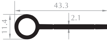
CERMAN MENTEŞE DÜZ HINGE PROFILE Kod/Code :MB1009 Ağırlık/Weight:0,313 kg/m
