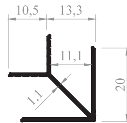
TAŞ GİRİŞ KÖŞE PROFİLİ CORNER PROFILE Kod/Code : CE1413 Ağırlık/Weight : 0,225 kg/m
