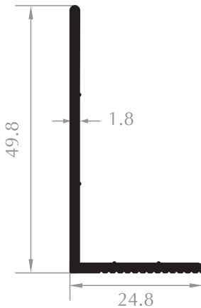
TIRTIKLI L L PROFILE Kod/Code :CE1404 Ağırlık/Weight:0,350 kg/m
