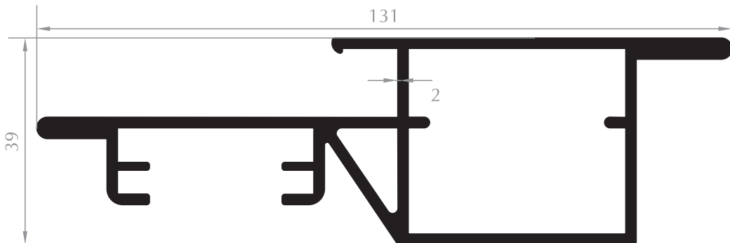
KAPI KASASI KISA DOOR FRAME Kod/Code :MH1968 Ağırlık/Weight: 2,002 kg/m
