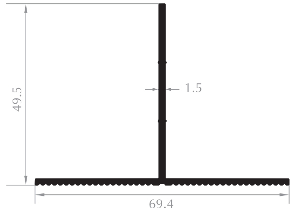
TIRTIKLI T T PROFILE Kod/Code :CE1407 Ağırlık/Weight:0,451 kg/m
