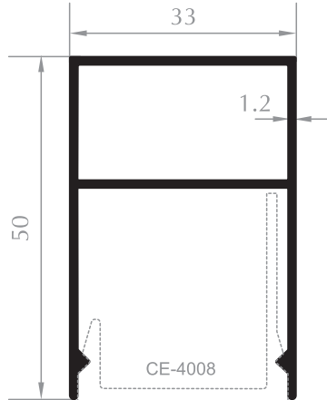
KAPAK PROFİLİ CAP PROFILE Kod/Code :CE4009 Ağırlık/Weight:0,544 kg/m
