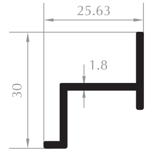
PERVAZ PROFİLİ SILL PROFILE Kod/Code :CE4031 Ağırlık/Weight: 0,286 kg/m
