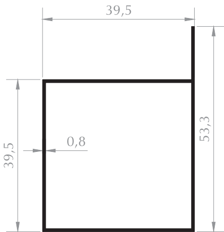
40x40 KULAKLI PROFİL 40x40 BOX PROFILE Kod/Code :MB1020 Ağırlık/Weight:0,365 kg/m
