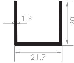
U PROFİLİ U PROFILE Kod/Code :DO1023 Ağırlık/Weight:0,209 kg/m
