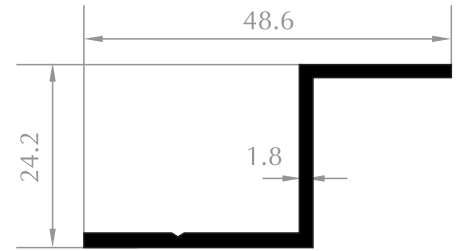
Z PROFİLİ Z PROFILE Kod/Code :CE4011 Ağırlık/Weight:0,336 kg/m
