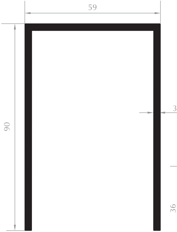
KOMPOZİT U PROFİLİ COMPOSITE U PROFILE Kod/Code : CE2504 Ağırlık/Weight: 1,895 kg/m
