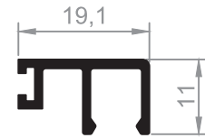
CAM ÇİTASI GLAZING BEAD
