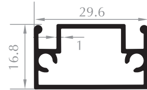
SİNEKLİK KANAT SASH PROFILE Kod/Code : SN1007 Ağırlık/Weight : 0,317 kg/m
