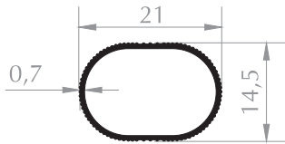
TIRTIKLI BORU PROFİLİ PIPE PROFILE Kod/Code : MB1008 Ağırlık/Weight : 0,116 kg/m
