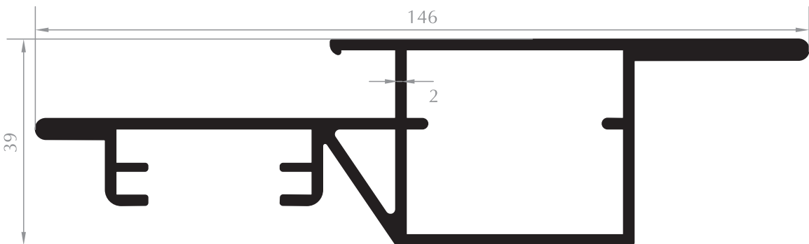
KAPI KASASI UZUN DOOR FRAME Kod/Code :MH1969 Ağırlık/Weight:2,165 kg/m
