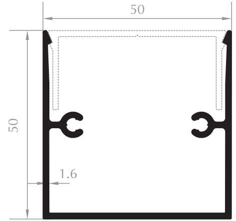
KAPAK PROFİLİ CAP PROFILE Kod/Code :CE4027 Ağırlık/Weight:0,769 kg/m
