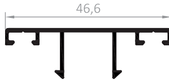
KAPAK PROFİLİ CAP PROFILE Kod/Code : OB-P03 Ağırlık/Weight : 0,260 kg/m
