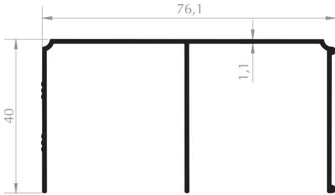
ÜST RAY PROFİLİ TOP RAIL PROFILE Kod/Code :MB3003 Ağırlık/Weight:0,577 kg/m
