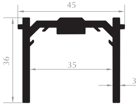
KOMPOZİT BAĞLANTI PROFİLİ COMPOSITE CONNECTION PROFILE Kod/Code : CE2505 Ağırlık/Weight: 1,056 kg/m
