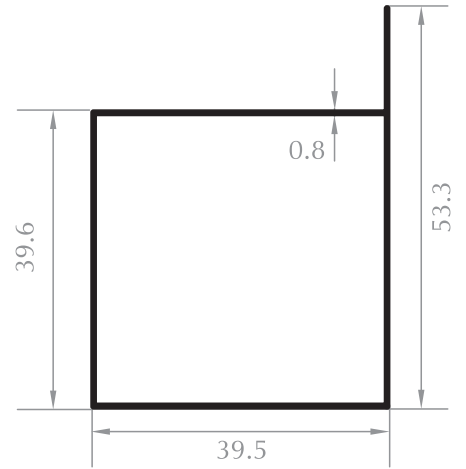
40x40 KUTU PROFİLİ 40x40 BOX PROFILE Kod/Code :MB1020 Ağırlık/Weight:0,365 kg/m
