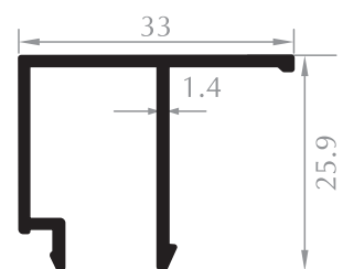
İSİ CAM ÇİTASI GLAZING BEAD Kod/Code :DO1018 Ağırlık/Weight:0,332 kg/m
