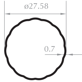
28'LİK SOBA BORUSU STOVE PIPE Kod/Code :MH1927 Ağırlık/Weight:0,160 kg/m
