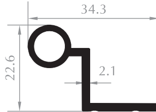
MOBİLYA MENTEŞE HINGE PROFILE Kod/Code :MB1010 Ağırlık/Weight:0,340 kg/m
