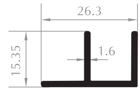
F PROFİL F PROFILE Kod/Code :CE4030 Ağırlık/Weight: 0,230 kg/m
